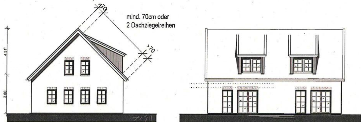
Abbildung 3: Dachgauben Dachziegelabstand
