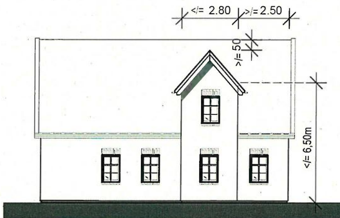
Abbildung 4: Dachkerker
